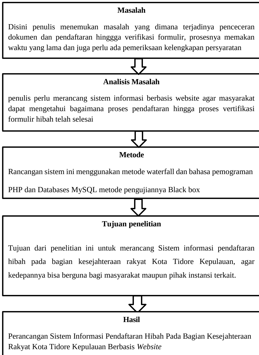
Gambar 2.2 Kerangka Berpikir
